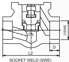
SOCKET WELD (SWE)
